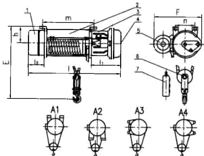
Рис.8 - Электрическая таль MD1 0.5 - 5 т, 6 - 36 м с жестким креплением
