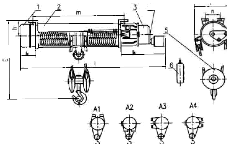
Рис. 12 - Электрическая таль MD1 10-20 т, 6-30 м с жестким креплением 1. редуктор скорости подъемного механизма; 2. наматывающий барабан; 3. двигатель для перемещения в вертикальной плоскости; 4. регулятор тормоза; 5. подъемный крюк; 6. пульт
