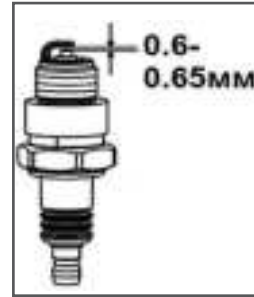
Рис.19 Свеча зажигания
