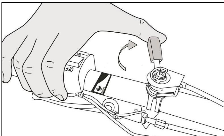
Рис. 30. Установка рычага газа в минимальное положение
