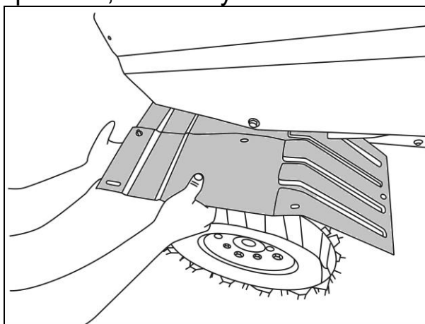
Рис. 10. Установка крыльев
