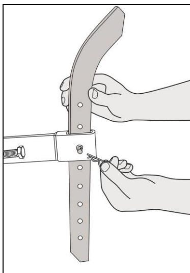
Рис.12. Установка сошника
