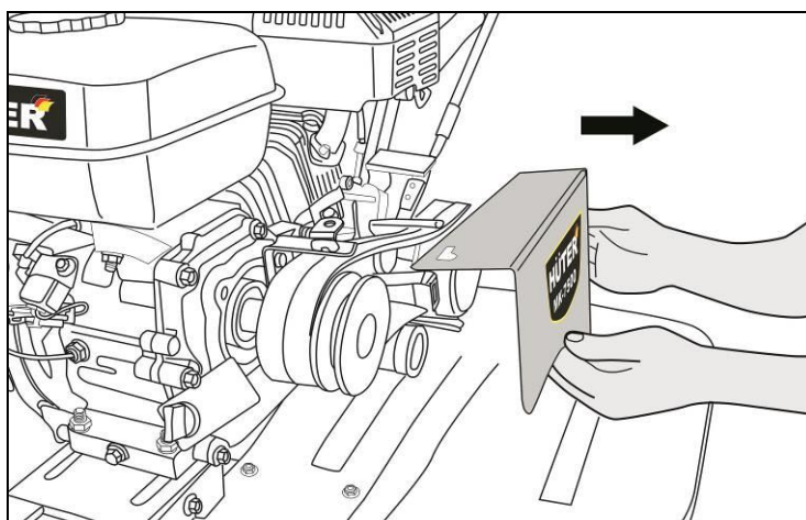
Рис. 34 Снятие защитной крышки
