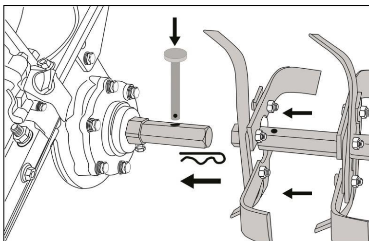
Рис. 8. Установка фрезы
