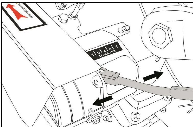
Рис. 26. Переключение скоростей коробки передач
