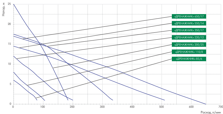
График расходно-напорных характеристик насосов серии «ДРЕНАЖНИК»
